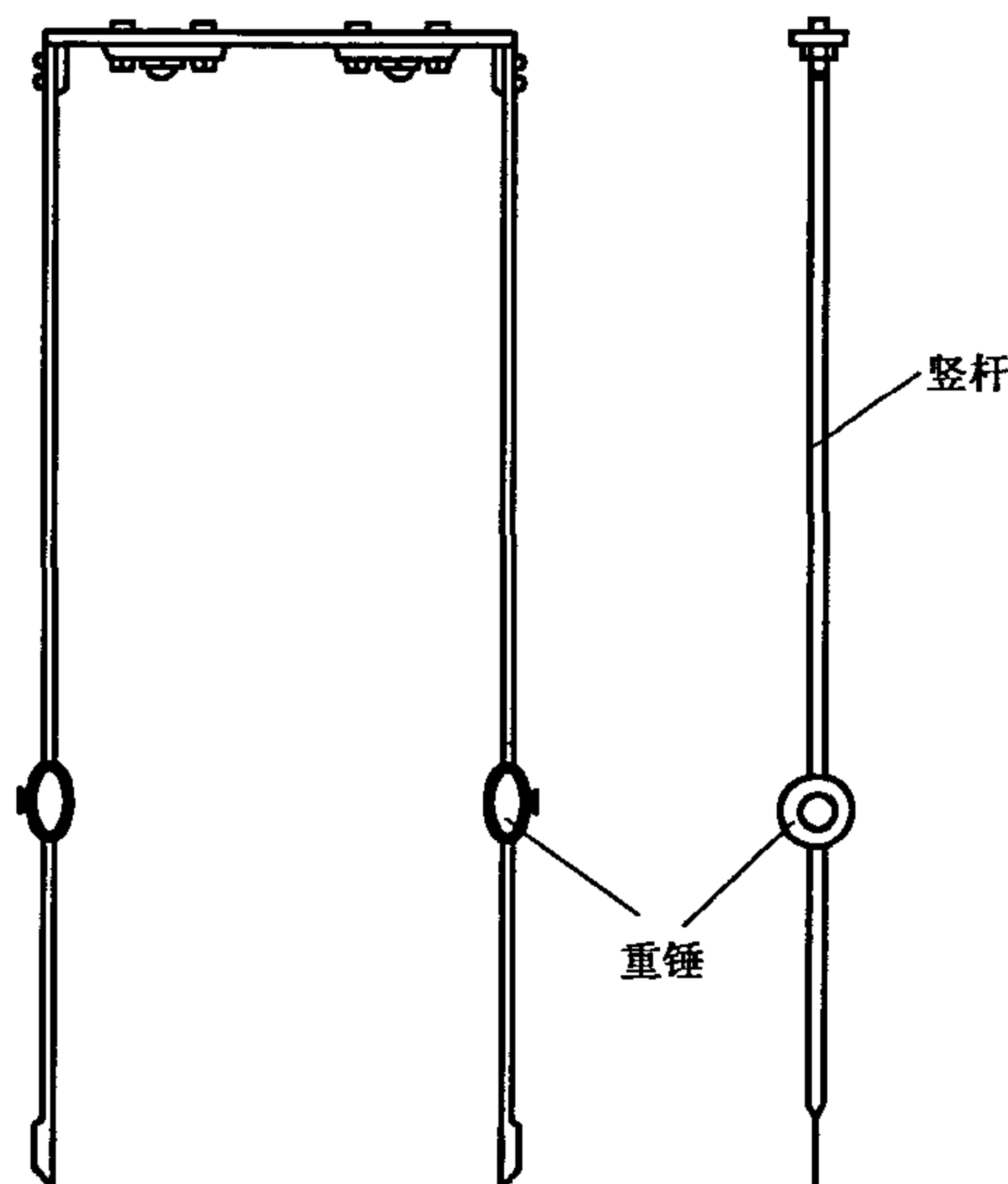
图 3 双摆
